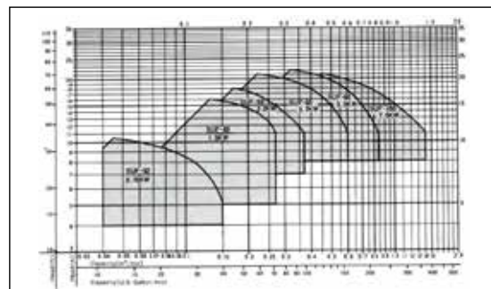
Model : SUF - (G) Motor speed : 2,880 r.p.m.
