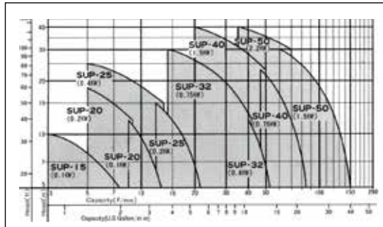
Model : SUP - (G) Motor speed : 1,450 r.p.m.
